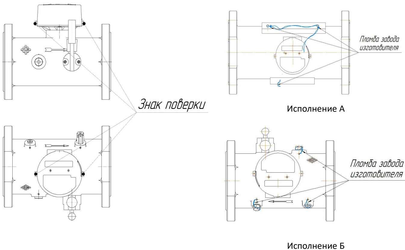
Схема пломбировки
